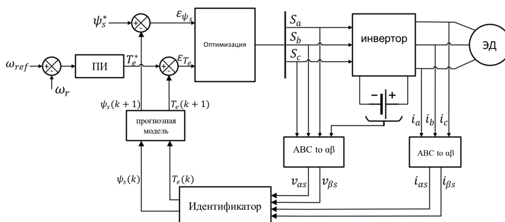
Рисунок 8 - Структурная схема Прямое управление моментом на основе прогнозирующей моделью.
